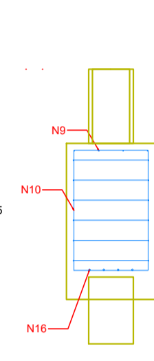
CORTE B-B ESC 1:25
