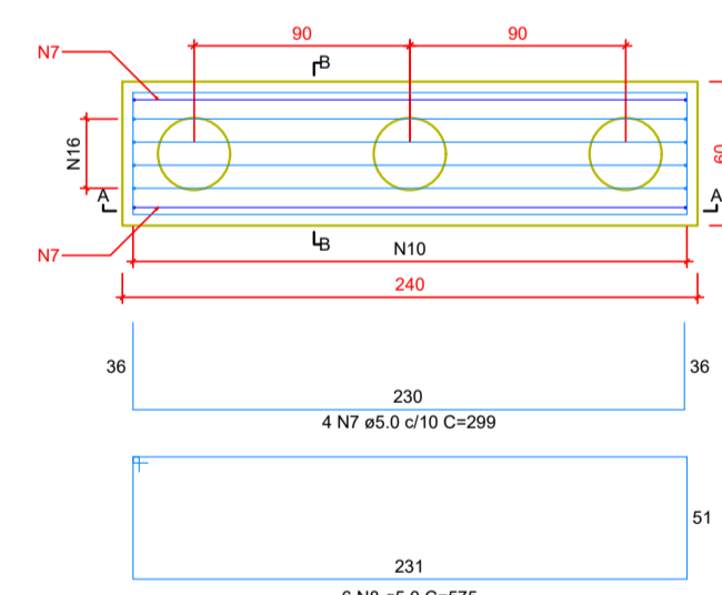
B18-19 3xC30 PLANTA ESC 1:25
