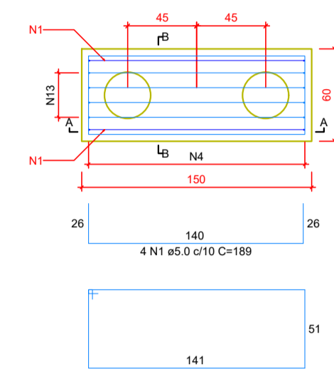
B6=B7=B35=B36 2xC30 PLANTA ESC 1:25
