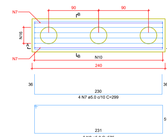
B22-23 3xC30 PLANTA ESC 1:25
