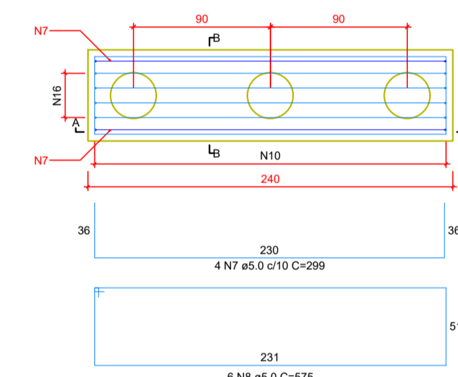
B16-17 3xC30 PLANTA ESC 1:25
