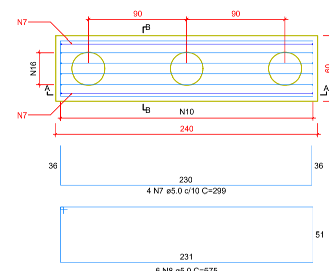
B12-13 3xC30 PLANTA ESC 1:25
