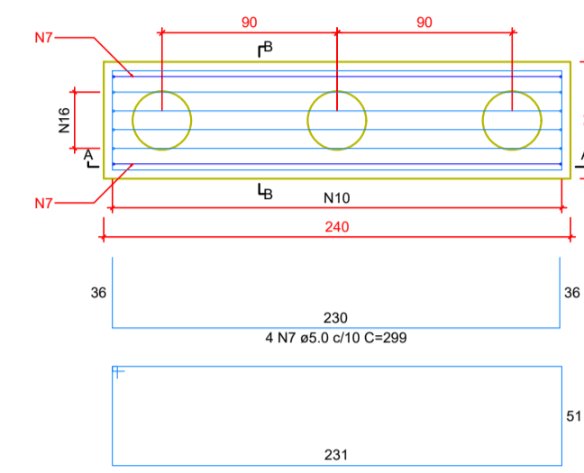
B10-11 3xC30 PLANTA ESC 1:25
